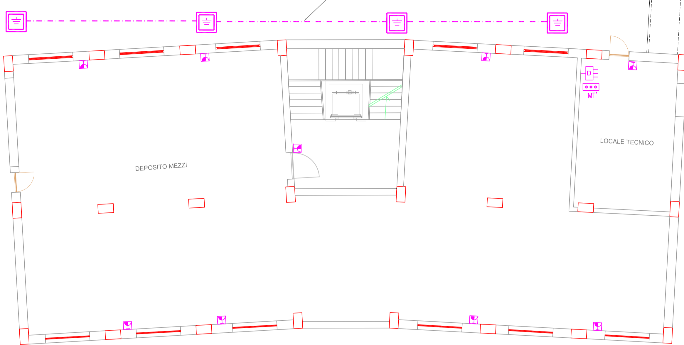
PIANTA PIANO SOTTOSTRADA
